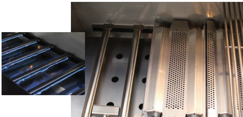
« BRIQUETTE SYSTEM WITH HYBRID BURNERS
